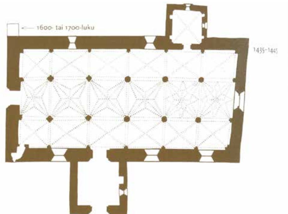
Pernajan kirkon pohjapiirustus ja osien ajoitukset Markus Hiekkasen mukaan. Piirustus: Markus Hiekkänen, teoksesta Hiekkänen 2014, 451.
