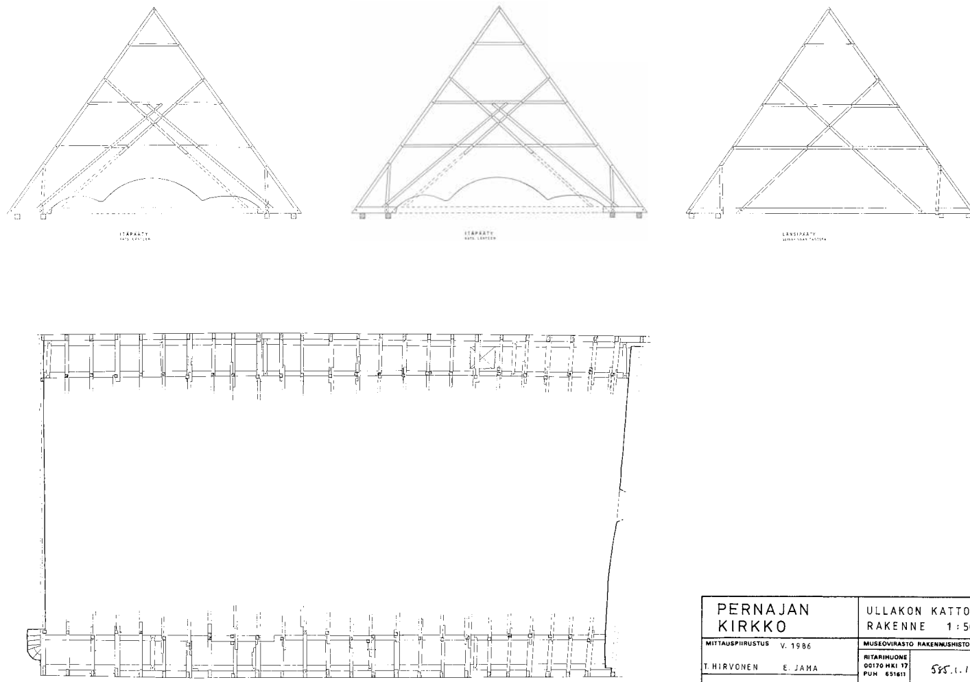
Pernajan kirkon ullakon kattotuolirakenteiden mittauspiirustukset vuodelta 1986. T. Hirvonen & E. Jama, Museoviraston rakennushistorian osasto. Säilyttävä arkisto: Museoviraston arkisto.
