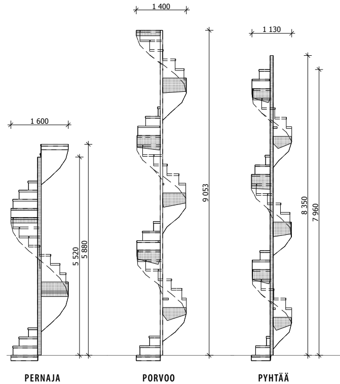
Pernajan, Porvoon ja Pyhtään kirkkojen ullakonportaat.
