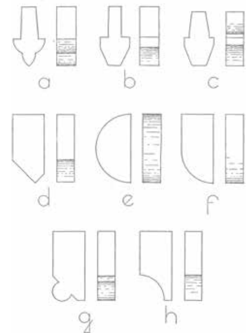
Pernajan kirkon eri rakennusosissa käytettyjä tiilityyppejä:
