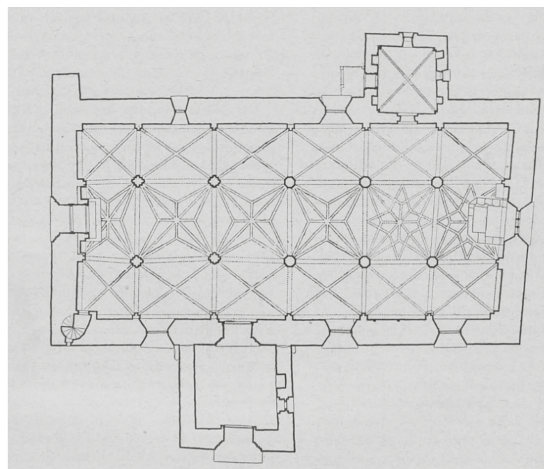
Pernajan kirkon leikkaus ja pohjapiirustus. Leikkauksessa ei ole esitetty savupiippuja, vaikka ne vielä vuonna 1926 olivatkin olemassa. Piirustukset: Arkkitehti-lehti numero 6, 1.1.1926, s. 79.
