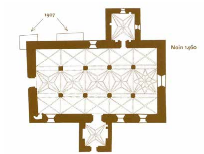
Pyhtään kirkon pohjapiirustus ja ajoitus Markus Hiekkasen mukaan. Piirustus: teoksesta Hiekkanen 2014, 464.
