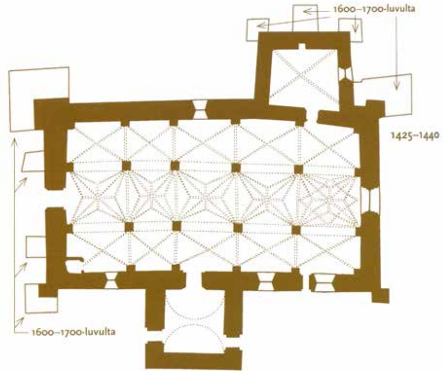
Varsinais-Suomessa sijaitsevan Taivassalon kirkon pohjapiirustus ja ajoitus Markus Hiekkasen mukaan. Taivassalon kirkkoon tehtiin alun perin puinen katto (laakea, lautainen segmenttiholvi) ja vasta myöhemmin päätettiin tehdä tiiliholvaus ja seiiniin rakennettiin tukipilarit. Piirustus: teoksesta Hiekkänen 2014, 176.
