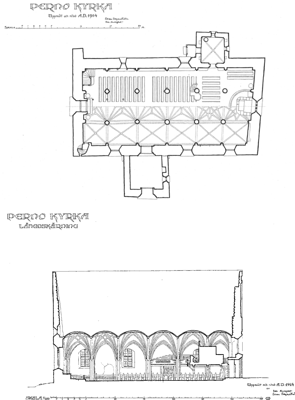
Pernajan kirkon piirustukset vuodelta 1914. Ellen Segerstråle ja Eva Kuhlefelt. Säilyttävä arkisto: Museoviraston arkisto.
